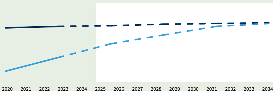
FIGURA 11. Dati di training utilizzati degli attuali modelli di IA vs stock di dati disponibili (numero di tokens - scala logaritmica), 2020 - 2024 (actual) 2025 - 2034 (forecast).
