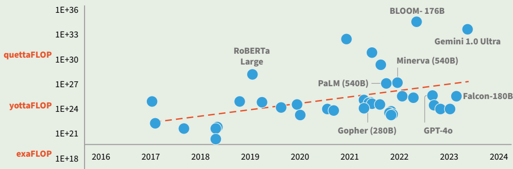
FIGURA 12. Risorse computazionali utilizzate per l'allenamento dei principali modelli di IA (FLOP - scala logaritmica), 2016 - 2024.
