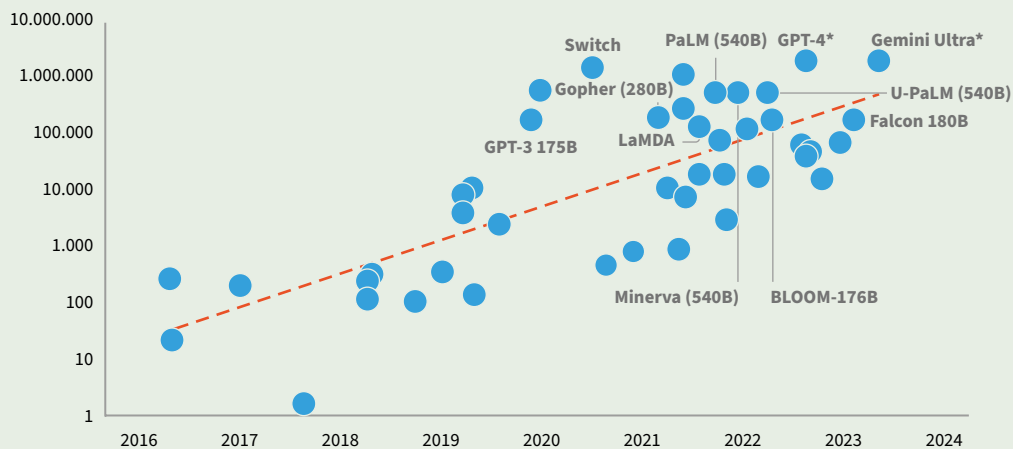
FIGURA 9. Numero di parametri dei principali modelli di IA (in milioni - scala logaritmica in base 10), 2016 - 2024.
