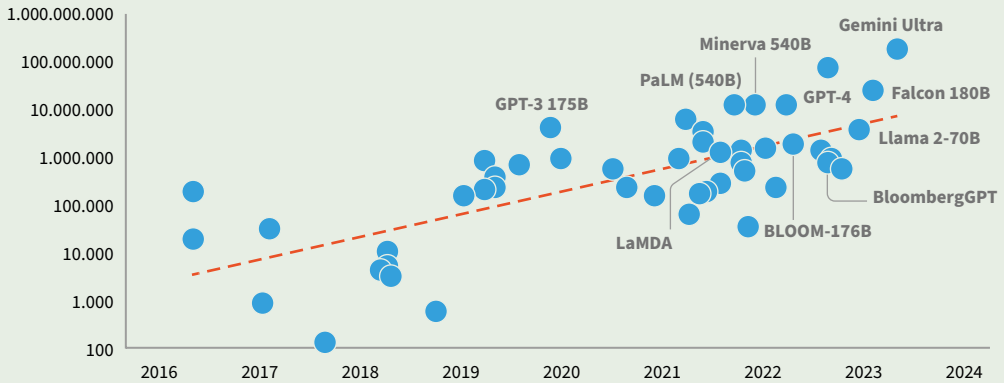
FIGURA 13. Investimenti per training dei principali modelli di IA (dollari - scala logaritmica), 2016 - 2024.
